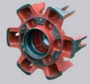
Spider B P W 16 T 604 202 224
